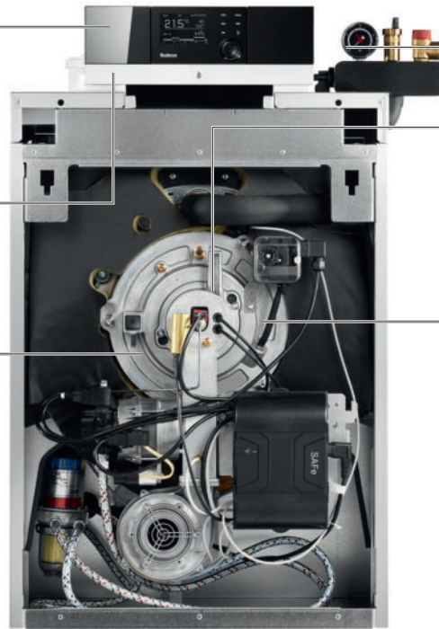
Logano plus KB195i BZ 19 kW & 25 kW
