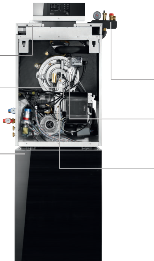
Logano plus KB195iT BZ
